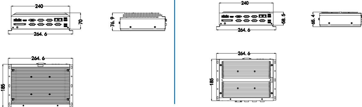
(具体配置尺寸, 见说明书) (单位: MM)
